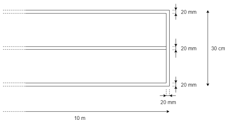
Figura 5: Detalhe das marcações de cada faixa de rodagem da pista de competição
