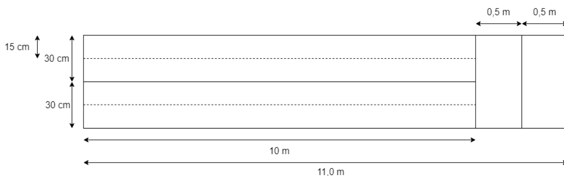
Figura 4: Dimensões aproximadas da pista de competição (figura não à escala)
